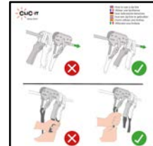
DAS432-9 « How to use a pulley »
