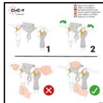
DAS432-8 « Como utilizar una polea C-ZIP »
